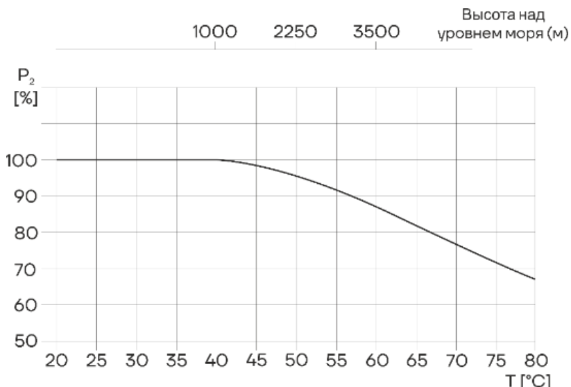
Рис. 5 Зависимость мощности электродвигателя от температуры/высоты над уровнем моря
