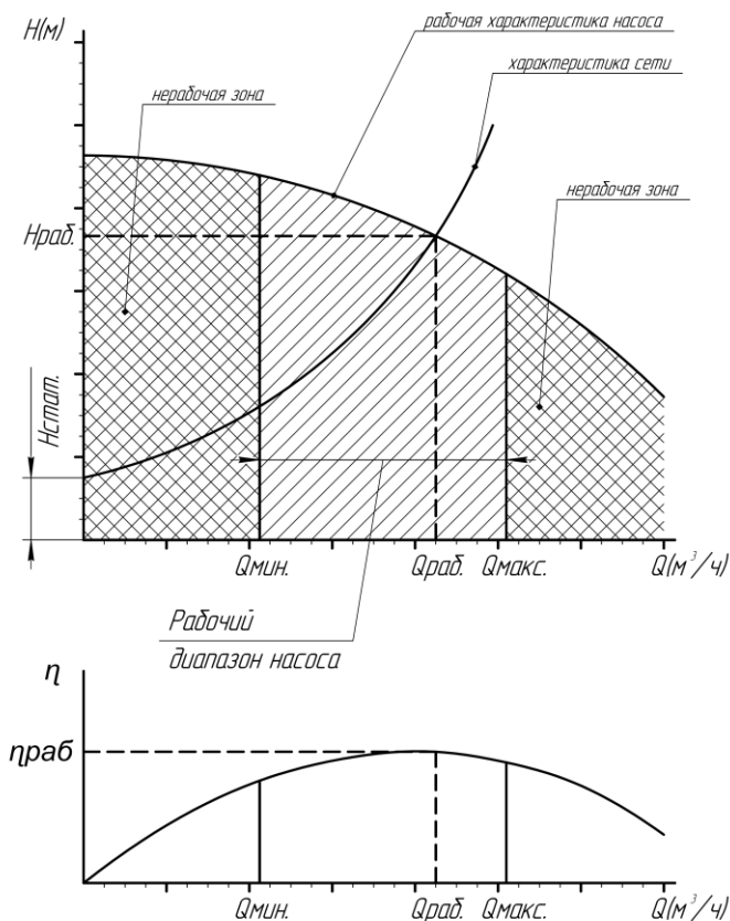
Рис. 6 Определение рабочей зоны насоса
