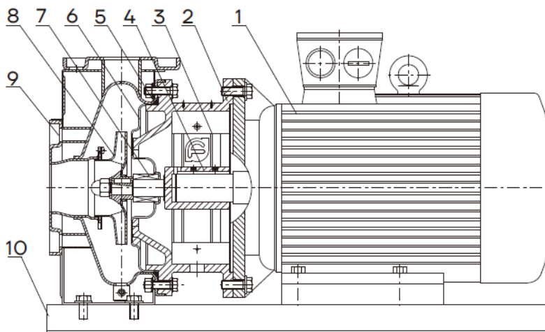
Рис. 4 Вид в разрезе ZS
