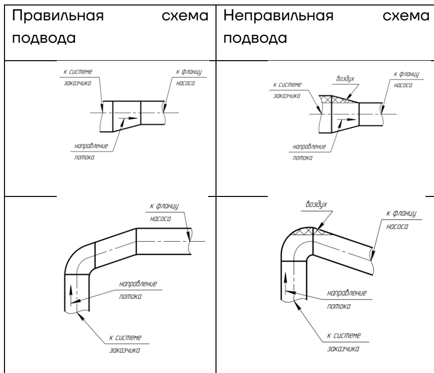
Рис. 9 Схемы подвода
