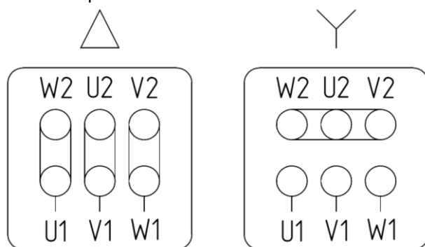
Рис. 11 Схема клеммных соединений
