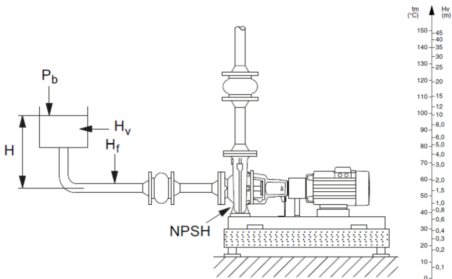
Рис. 7 Система с насосом
