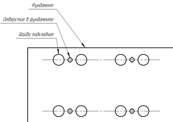
Рис. 8 Схема расположения шайб на фундаменте (вид сверху)
