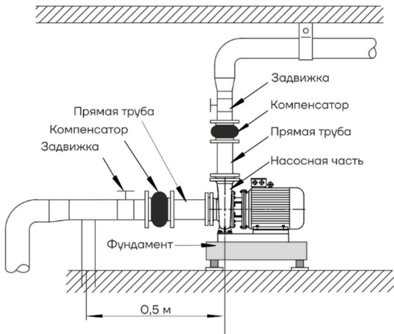
Рис. 10 Рекомендуемая схема подключения
